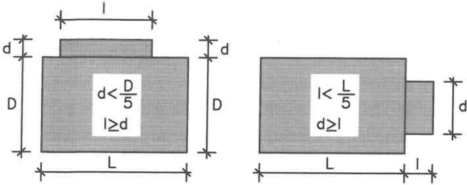
الف) پیش‌آمدگی در امتداد طول ساختمان ب) پیش‌آمدگی در امتداد عرض ساختمان شکل ۱-۷ ابعاد پیش‌آمدگی در پلان ساختمان
