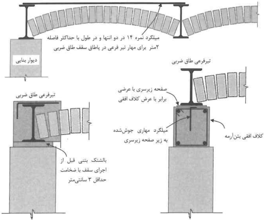
ب- ترکیب تیرفرعی باطاق یا کلاف افقی
